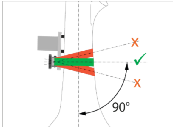
Kuva 4: Kiristyshihnan oikeanlainen asennus
