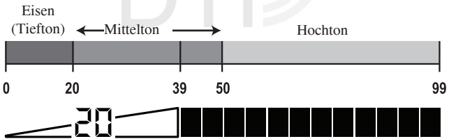
IRON AUDIO AN: Metallobjekte unterhalb 20 werden mit Tief-Ton hörbar und oberhalb mit Mittel- oder Hochton hörbar gemacht.
